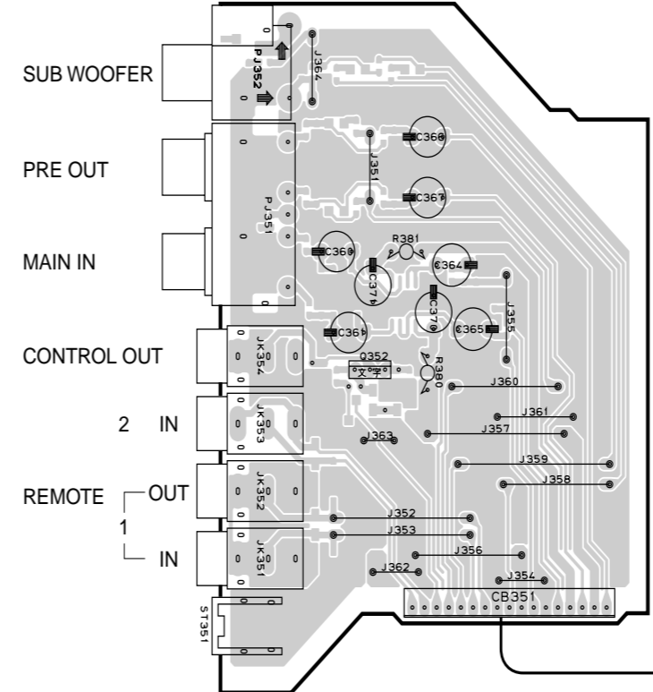
FUNCTION (4) P.C.B. (Side A)
