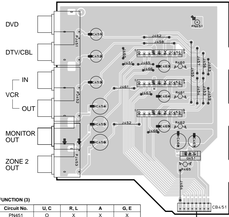
FUNCTION (3) P.C.B. (Side A)
